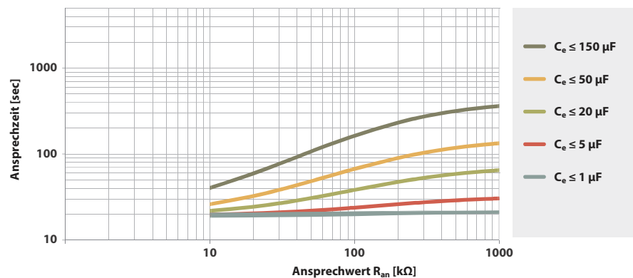
Ansprechzeit in Abhängigkeit vom Ansprechwert und der Netzableitkapazität nach IEC 61557-8 ( U_n = AC\ 690\ V , f_n = 60\ Hz )
